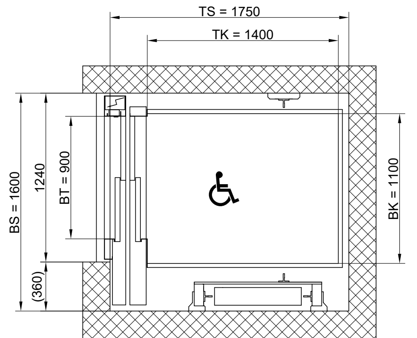
Nutzlast 630kg / 8 Pers. Türen rechtsöffnend
