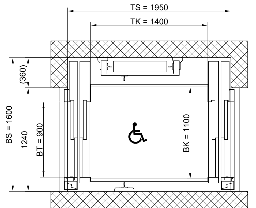
Nutzlast 630kg / 8 Pers. Türen gegenüberliegend
