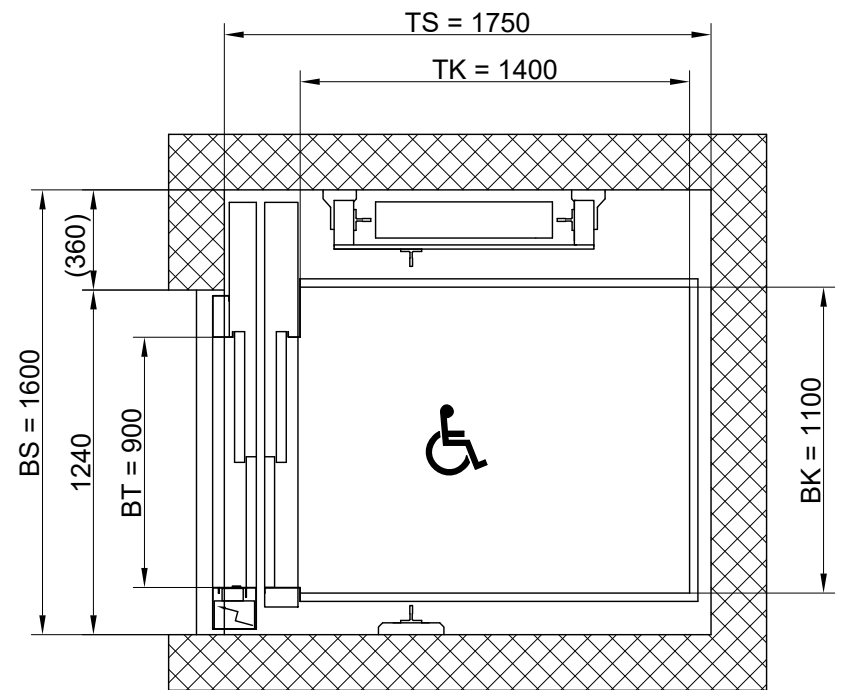
Nutzlast 630kg / 8 Pers. Türen linksöffnend
